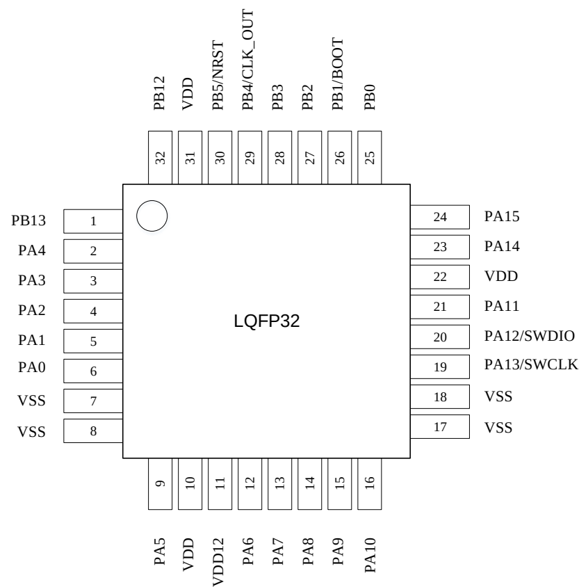
图 1-2 LQFP32 封装管脚分布图
