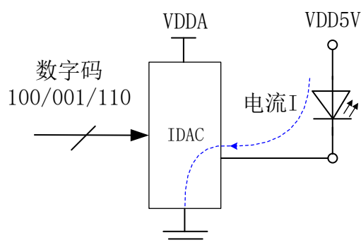
IDAC 的典型应用电路
